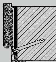
Muuromvattend kozijn Diagonale bevestiging tot muurdikte 175
