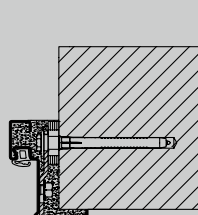
Hoekkozijn met verdoken plugmontage
