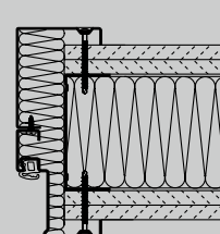
Hoek- en tegenkozijn Schroefmontage
