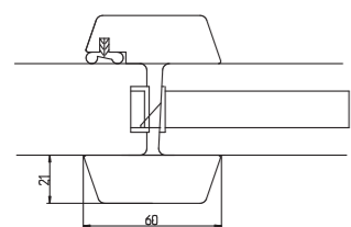
Aanslaglatten incl. driepuntsluiting en sluitlijst.
