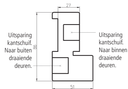
Tongstijl eventueel met uitsparing tbv kantschuif.
