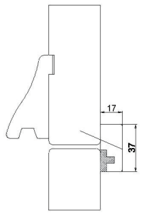
Standaard duo doorsnede
