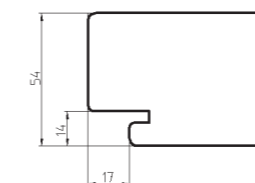
kader profiel 17 mm
